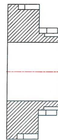
B-B (1:1,5)
